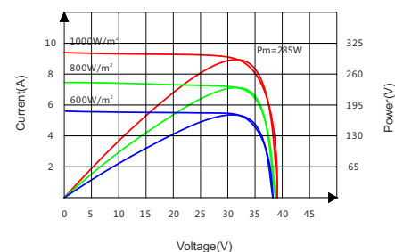
Current-Voltage&Power-Voltage Curve(285W)
