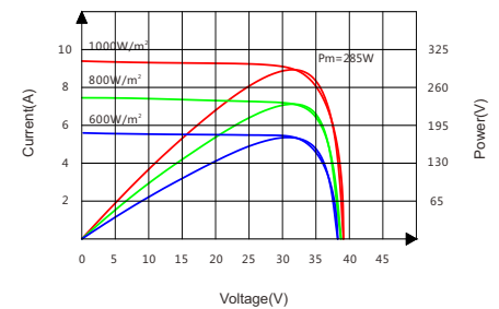
Current-Voltage&Power-Voltage Curve(285W)
