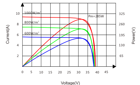
Current-Voltage&Power-Voltage Curve(285W)
